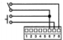
Botão do Retorno ou dispositivo NPN
