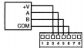
Gerador de pulsos por quadratura
